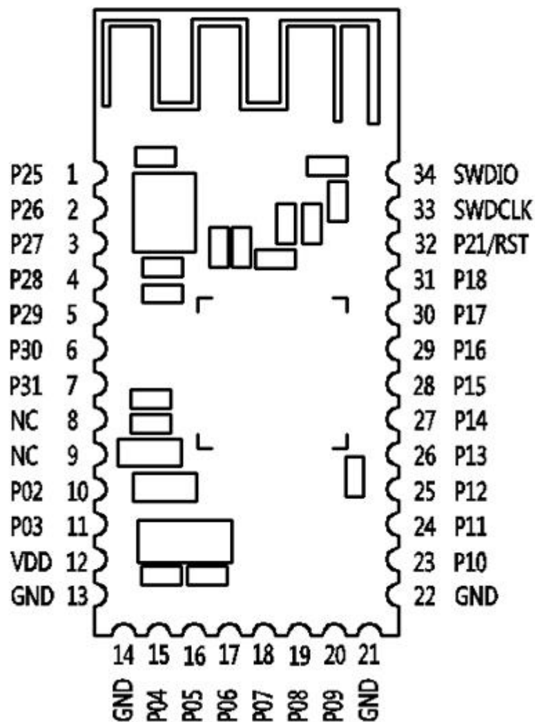
管脚布局 (仰视图)
