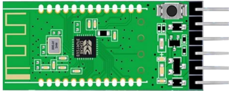
D32蓝牙模块（带底板）
