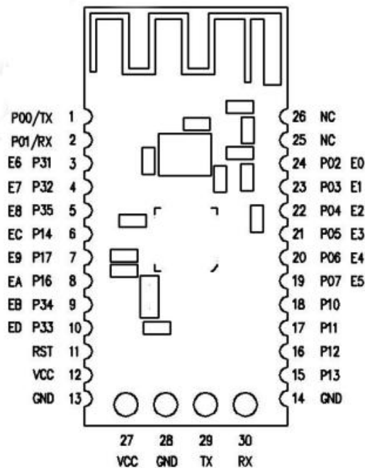
引脚映射图
