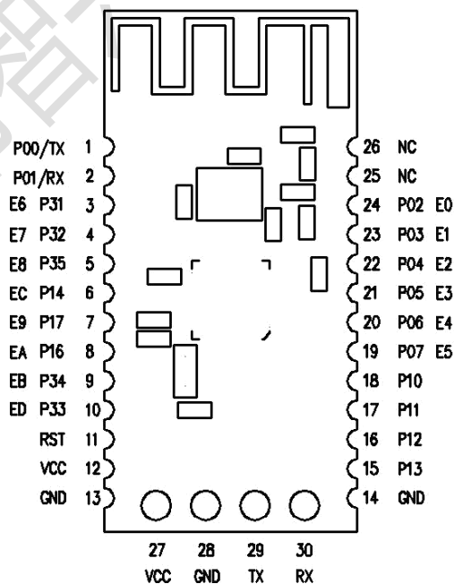
引脚映射图
