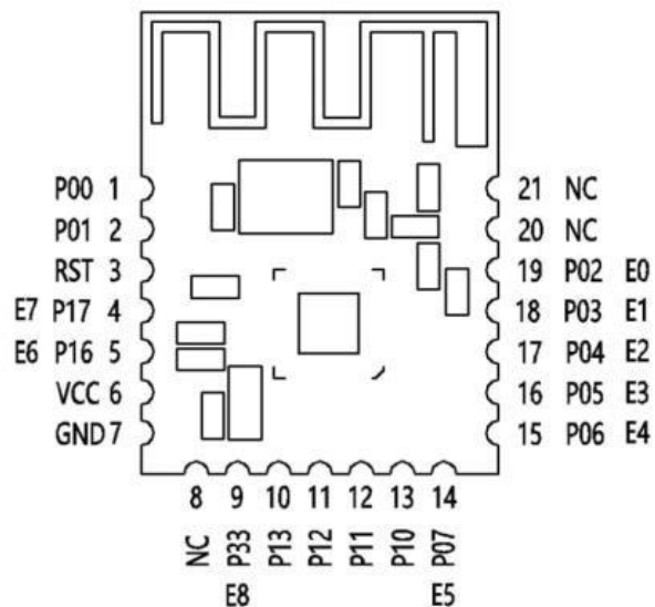
引脚映射图
