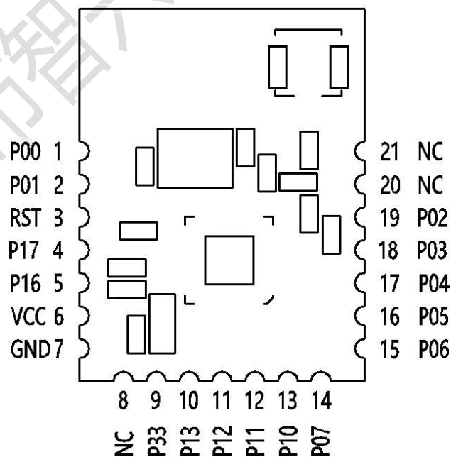
引脚映射图
